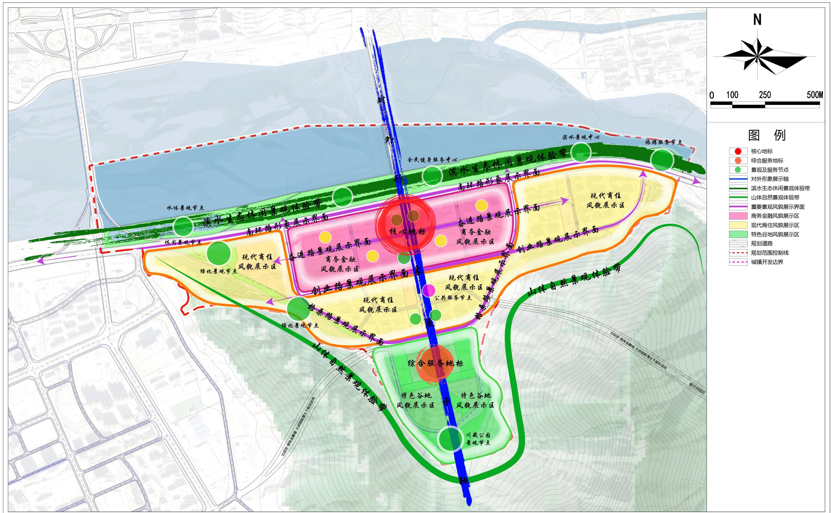
城市设计总体结构图
